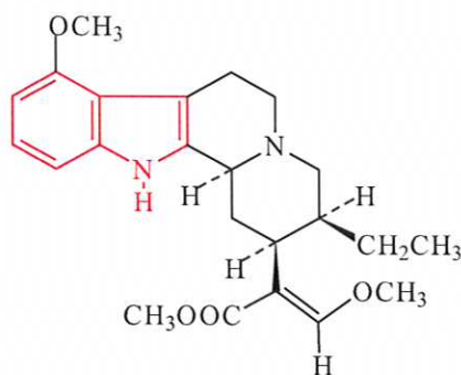
Mitragynine C_{23}H_{30}N_2O_4 MW : 398.5
